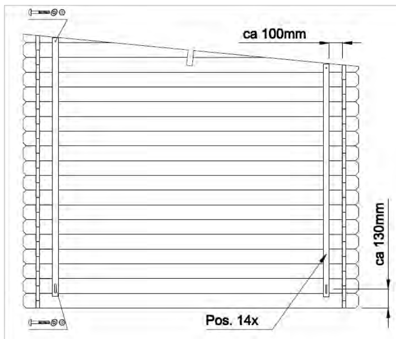
Установка штормовых планок:
