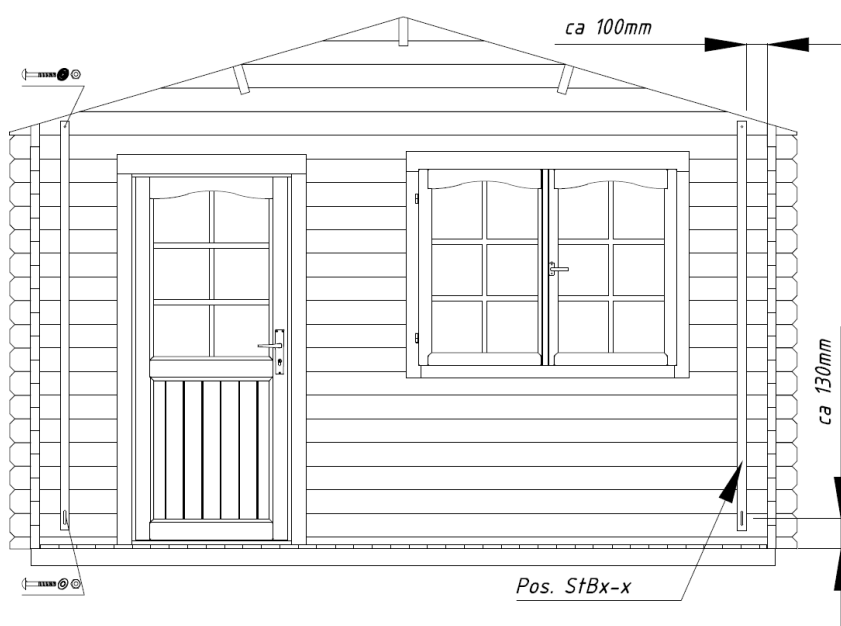
Tormiliistude paigaldus:
